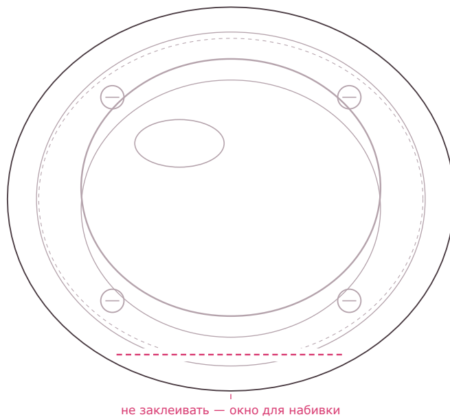
Деталь 1 — лицевая
